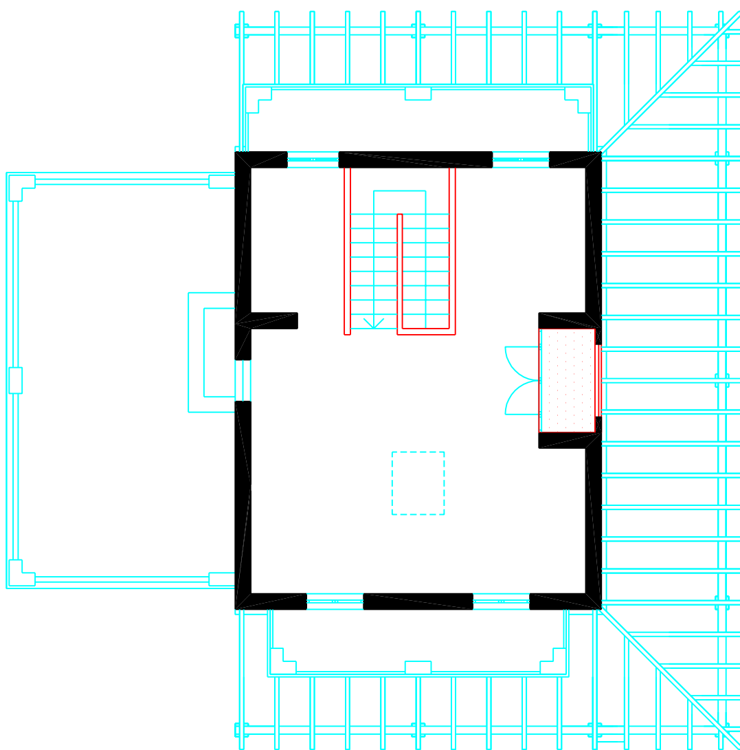
Pianta Mansarda scala 1:100
